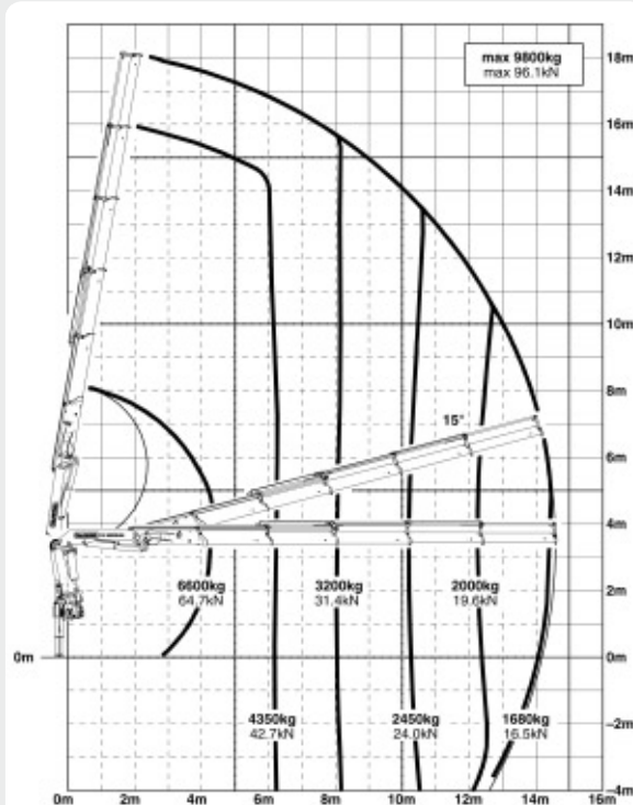
Grue 33-mto
