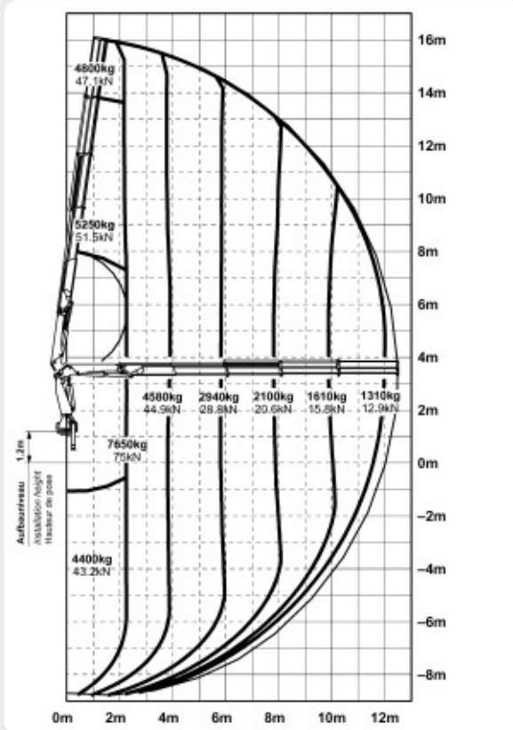
Grue 21-mto
